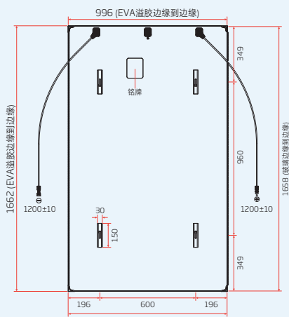
后视图 (横装)
