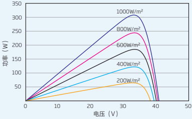
组件的P-V曲线 (305W)
