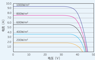
组件的I-V曲线(335W)
