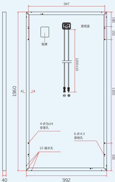
组件尺寸 (mm)
