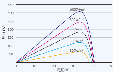
PVモジュール (305W) の P-V 曲線
